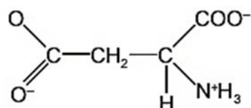
aspartate
